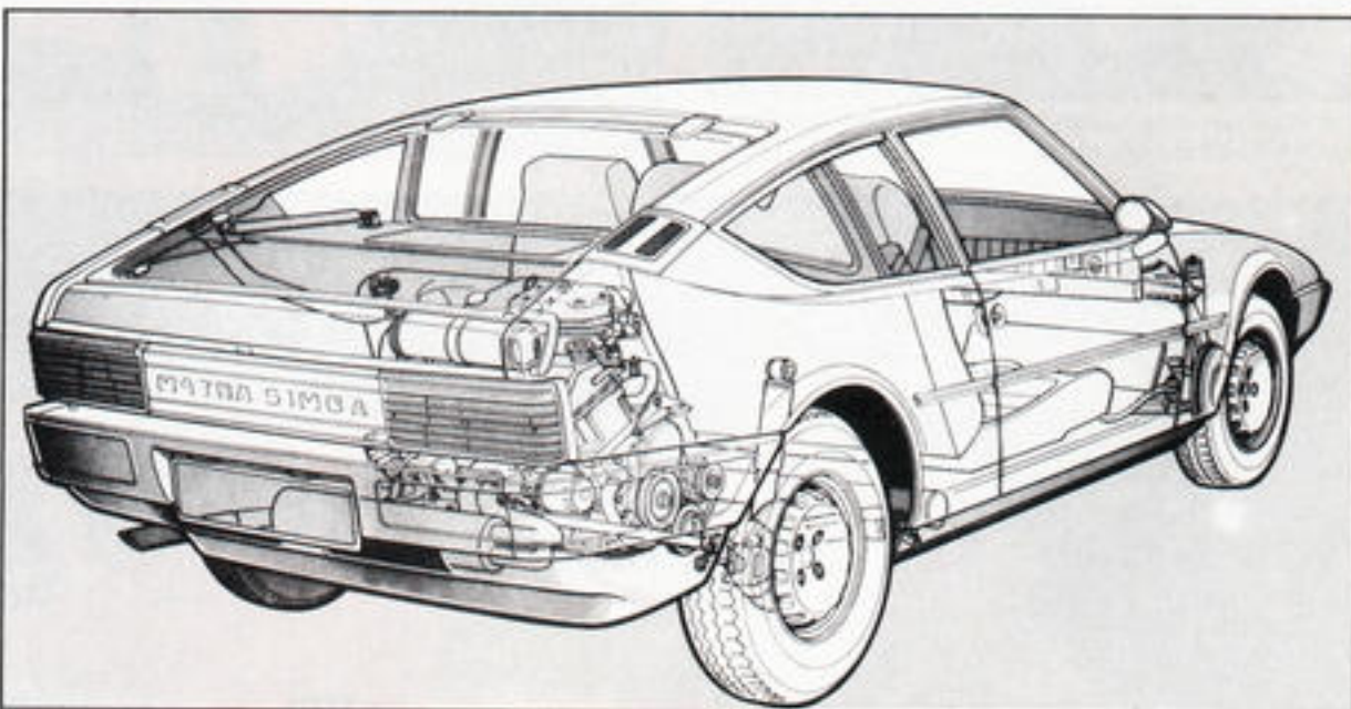
Der Mittelmotor bescherte eine erstaunliche Straßenlage, aber auch genauso viele Wartungsprobleme.
