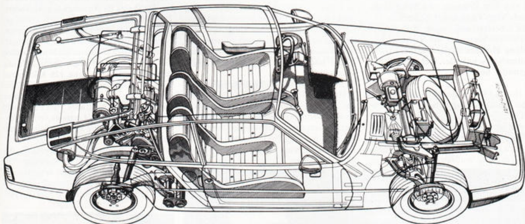
Das Röntgenbild zeigt die außergewöhnlichen Lösungen des Bagheera: drei nebeneinander angeordnete Sitze, Mittelmotor, rundum Scheibenbremsen, einzeln aufgehängte Räder.
